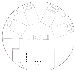
間取り図 (和洋室)
